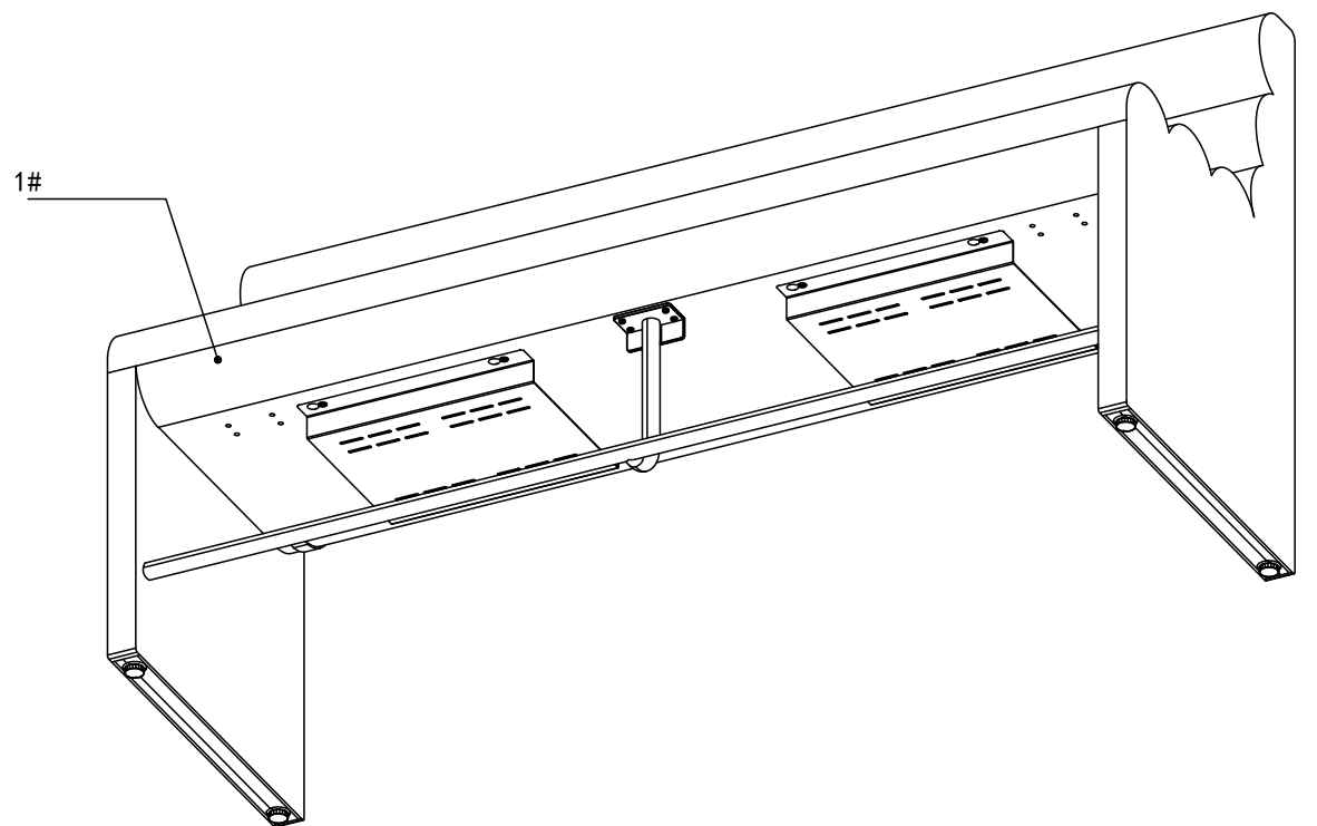
下面図 底部视角 Bottom view
