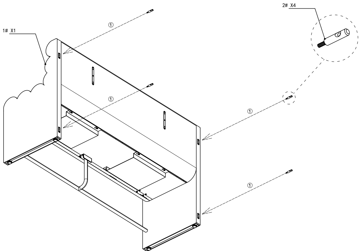
背面図 背面视角 Back view
