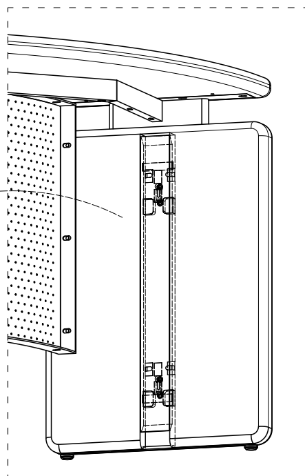
配線コードを入れたら、脚配線カバーを取り付けてください。 先将电线收进去，然后将这块板安装回去
