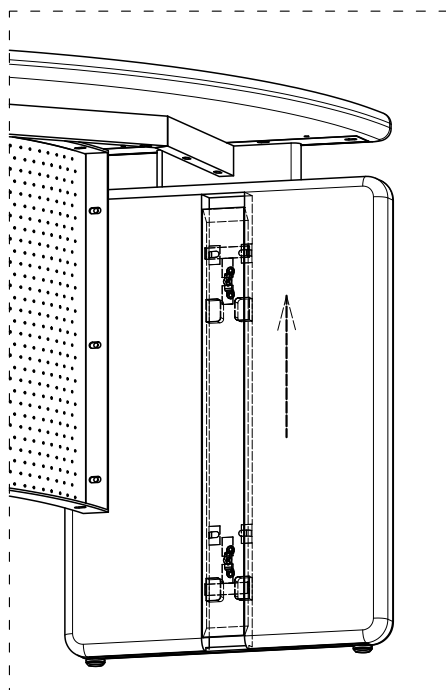
脚配線カバー 桌脚本身上面的过线盖 The wire cover on the top of the table leg itself
